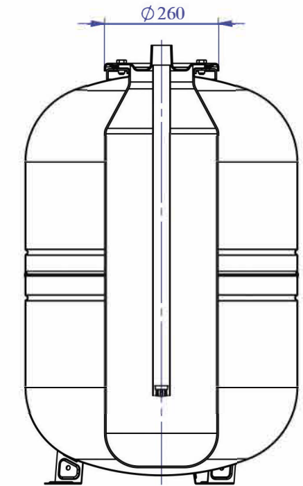
SEZIONE A-A
