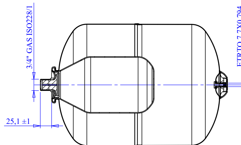
SEZIONE E-E
